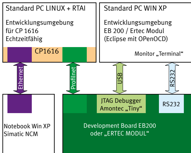
Abb. 1: Aufbau zur Untersuchung von Linux mit Echtzeiterweiterung und Profinet Kommunikation im Detail.
