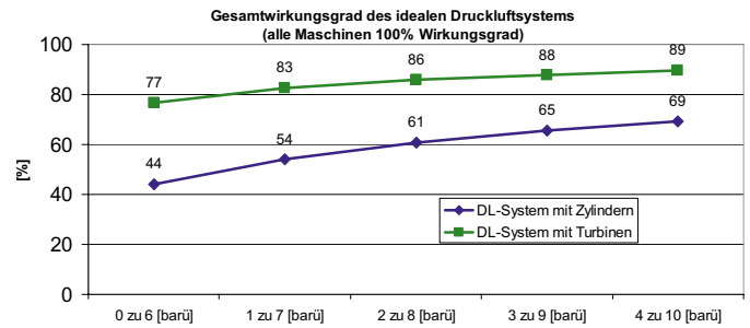
Abb. 8: Wirkungsgrad des Druckluftsystems als Funktion des Druckniveaus
