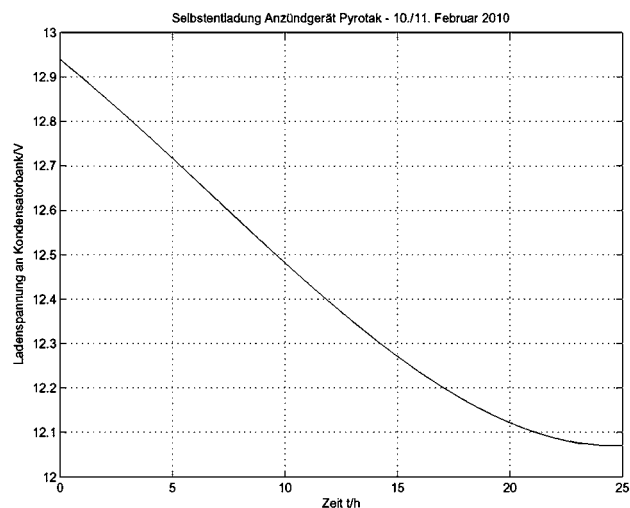
Abb. 4 Messung der Selbstentladung der C-Bank ohne Bordspannung
