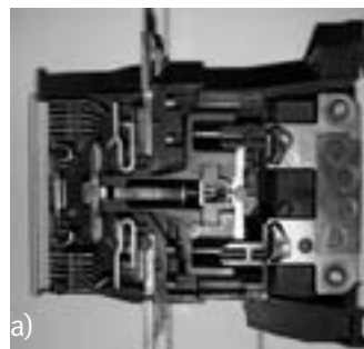
Abbildung 1: Schnittbilder a) Leistungs- und b) Leitungsschalter mit Löschblechen
