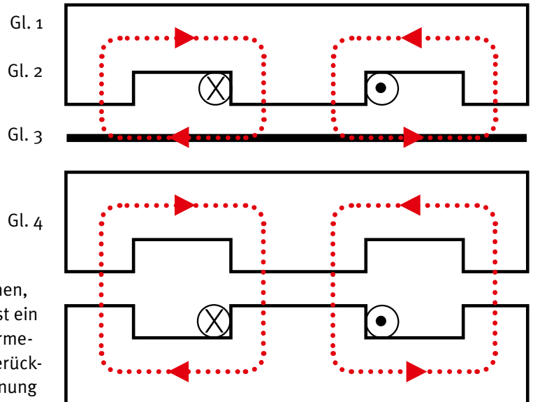
Abb. 4 a): prinzipieller Aufbau
