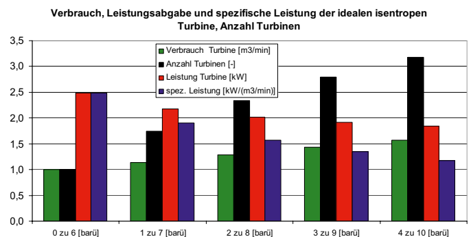
Abb. 6: Verbrauch, Leistungsabgabe und spezifische Leistung der Turbine, Anzahl der Turbinen als Funktion des Turbineneintritts- und -austrittsdruckes ( \Delta p_T = 6 \text{ bar} = \text{const.} ).
