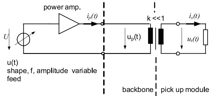
Abb. 3: Prinzipieller elektrotechnischer Aufbau
