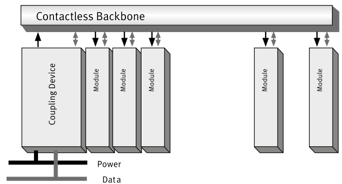
Abb. 1: Schematischer Aufbau der kontaktlosen Energie- und Datenübertragung
