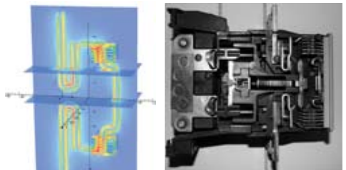
Abb. 4: Berechnete Magnetfeldverteilung und Schnittmodell des Schalters
