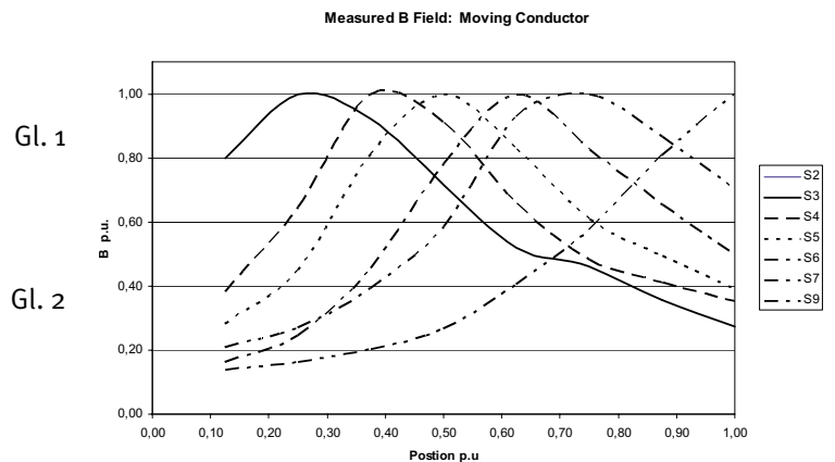
Abb. 3: Messwerte des ortsveränderlichen Magnetfeldes
