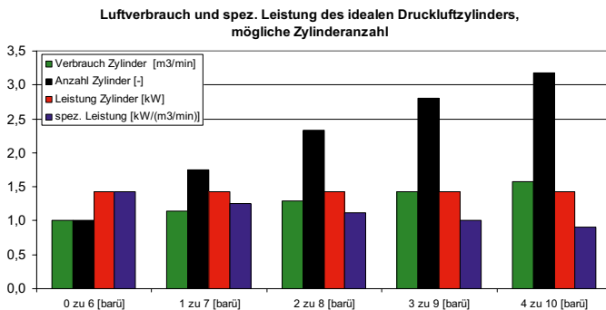
Abb. 4: Luftverbrauch und spez. Leistung des Zylinders, mögliche Zylinderanzahl als Funktion des Verdichtungsstartdruckes p_{\text{ein, K}} (hier Überdruck) bei festgehaltener Verdichtungsdruckdifferenz \Delta p = p_{\text{aus, K}} - p_{\text{ein, K}} = 6 \text{ bar} .
