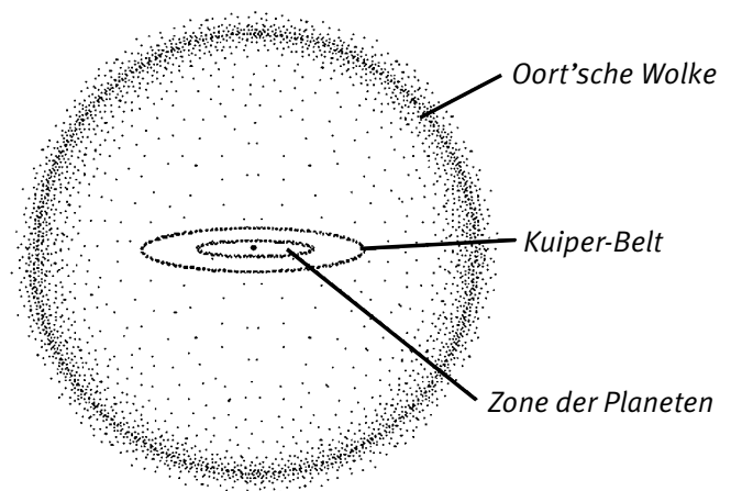
Abb. 2: Oort'sche Wolke (nicht maßstabsgerecht)
