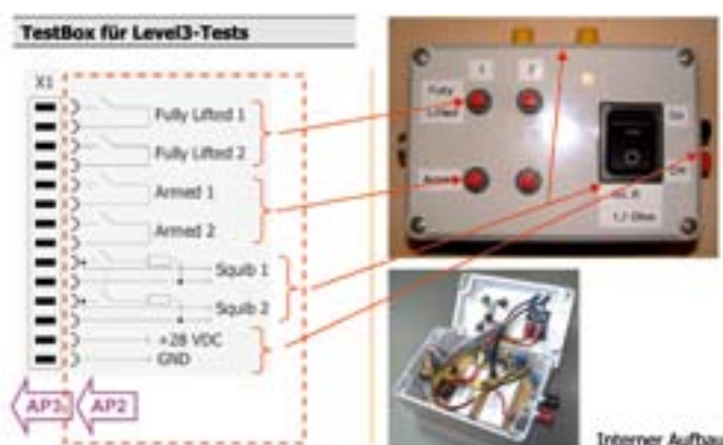
Abb. 3 TestBox mit Verdrahtungsplan
